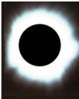
这是张日食时的照片，它证明了天地也可能被黑暗吞没
