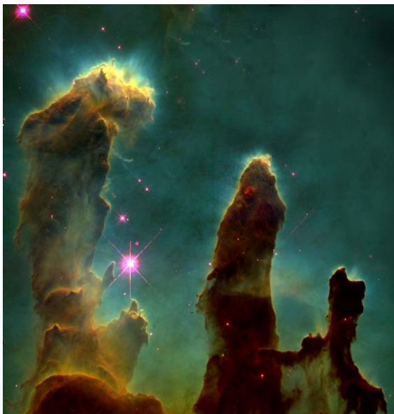
此图为一星球的实际图片,它已经成为星际物质
